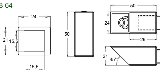
Glasanschluss ±90° verstellbar , für 6 - 10 mm Glasdicke und Stabilisierungsstange Art.-Nr. 47 360ff
