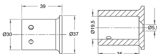
Wandanschluss 45^\circ , für Stabilisierungsstange Art.-Nr. 47 300ff
