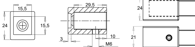
Wandanschluss verstellbar ±90° , für Stabilisierungsstange Art.-Nr. 47 360ff
