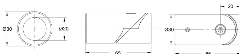
Wandanschluss, für Stabilisierungsstange Art.-Nr. 47 300ff
