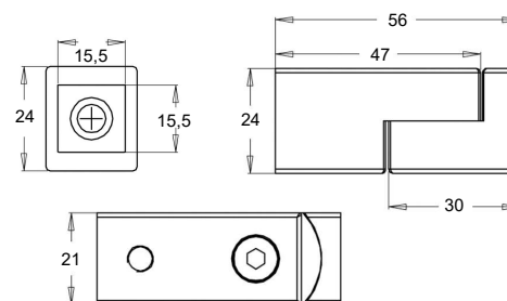
Wandanschluss verstellbar ±90° , für Stabilisierungsstange Art.-Nr. 47 360ff
