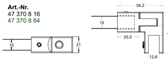
Glasanschluss ±90° verstellbar , für 6 - 10 mm Glasdicke und Stabilisierungsstange Art.-Nr. 47 360ff
