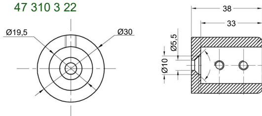
Wandanschluss verstellbar \pm 90^\circ , für Stabilisierungsstange Art.-Nr. 47 300ff
