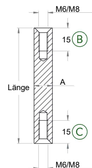
Stift, beidseitig Innengewinde, Edelstahl V2A 240 Korn geschliffen
