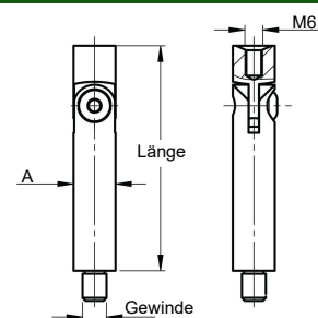
Gelenkstift, 1 x Außengewinde und 1 x Innengewinde M6
