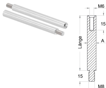
Stift, 1 x Außengewinde M8 und 1 x Innengewinde M6
