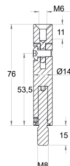
Gelenkstift Ø 14 mm (Winkel 0 - 59°) mit 1 x Innengewinde M6 und 1 x Außenwinde M8, Länge: 76 mm, 360° drehbar (mittels Klemmsystem durch seitliche Madenschraube beliebig am Pfosten ausrichtbar),
