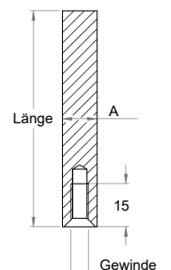
Stift, 1 x Innengewinde und 1 x flach, Edelstahl V2A 240 Korn geschliffen
