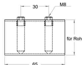
Rundrohr-Verbinder mit Klemmschrauben, zum Einstecken , Edelstahl V2A roh
