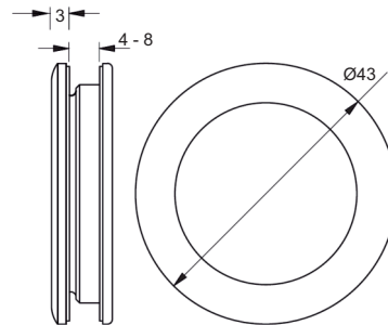
Glasbohrung Ø 37 mm
