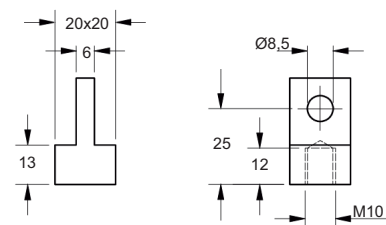
Gabel mit Stift und Sicherungsring, Edelstahl V2A geschliffet
