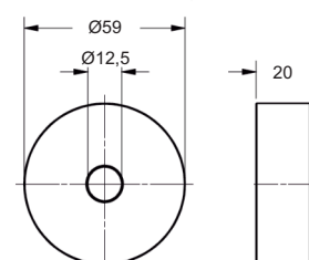
Distanzflansch für Wandbefestigung Art.-Nr. 55 410 8 00, Edelstahl V2A geschliffet
