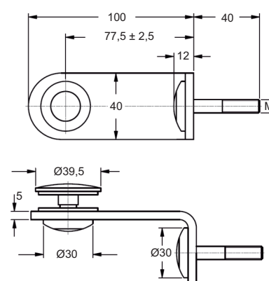
Punkthalter für 8 - 12 mm Glasdicke, mit Befestigungswinkel für Windfang-Set, Edelstahl V2A geschliffet
