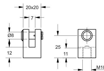
Gabel mit Stift und Sicherungsring, Edelstahl V2A geschliffet
