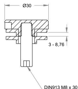
BRENK-fix® Oberteil Ø 30 mm für 3 - 8,76 mm Plattendicke, mit Gewindestift M8 x 30 mm
