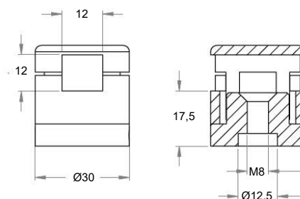
BRENK-fix® Grundhalter Ø 30 mm mit Innengewinde M8, für Stab 12 x 12 mm
