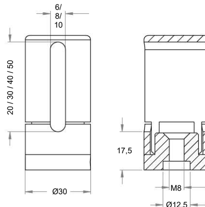
BRENK-fix® Oberteil Ø 30 mm für 3 - 8,76 mm Plattendicke, mit Gewindestift M8 x 30 mm
